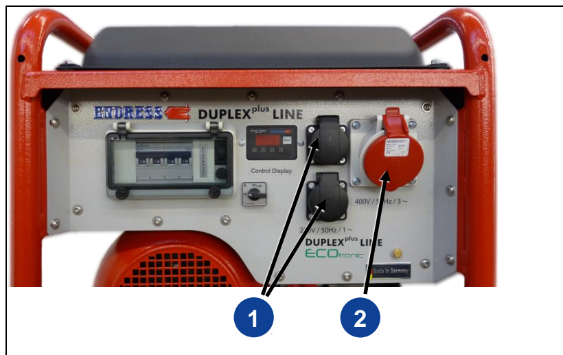
Abb. 4-5: Verbraucher anschließen
