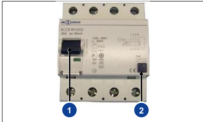
Abb. 5-1: FI-Schutzschalter
